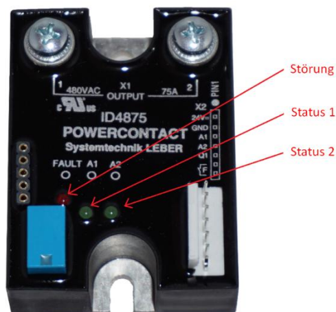
Abbildung 4: Status-LEDs
