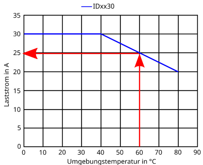
Abbildung 12: Beispiel zur Ermittlung des max. zulässigen Laststroms
