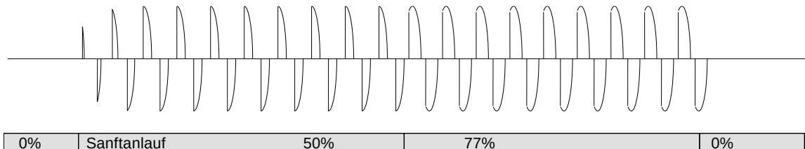
Abbildung 2: Darstellung des Phasenanschnitts
