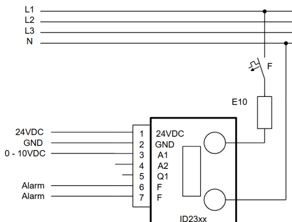
Abbildung 7: typischer Anschluss 230VAC
