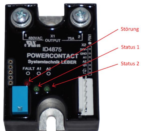
Abbildung 4: Status-LEDs
