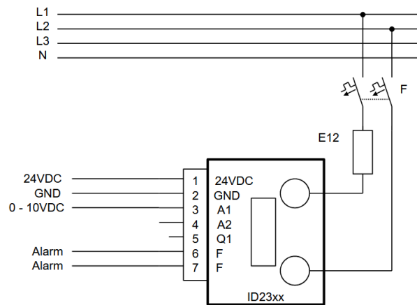
Abbildung 8: typischer Anschluss 400VAC
