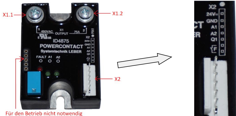
Abbildung 3: Belegung Stecker X1.1, X1.2 und X2
