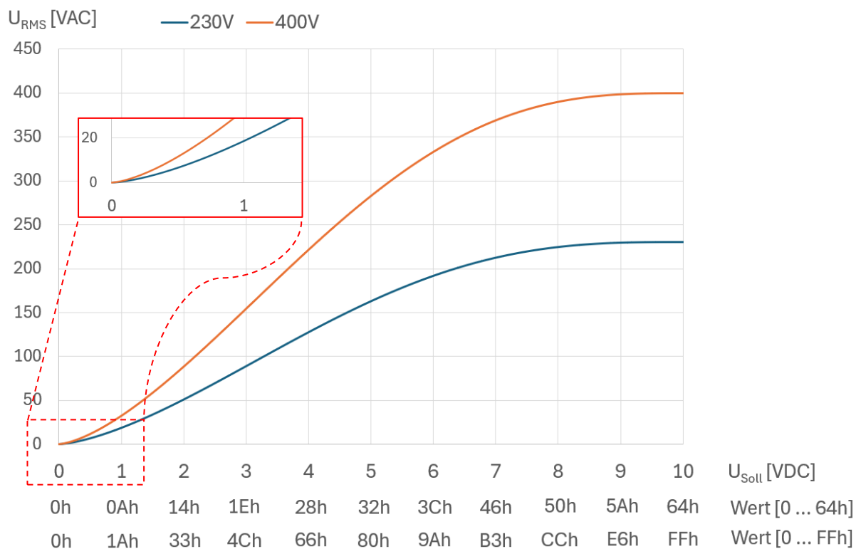
Abbildung 10: Effektive Lastspannung vs. Steuerspannung
