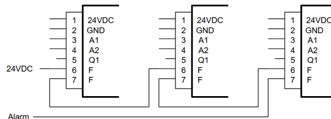
Abbildung 14: Ausführung mit Summen-Alarm-Auswertung
