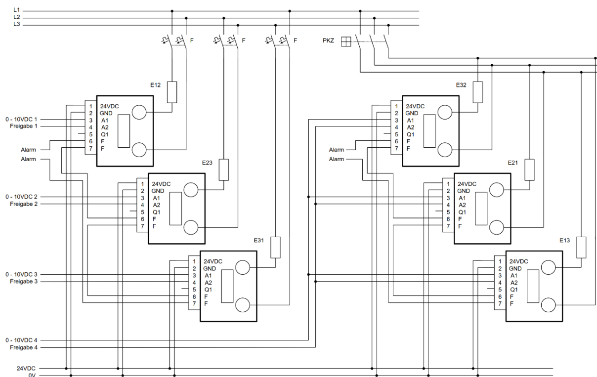
Abbildung 9: Darstellung von 3-phasen Anwendungen
