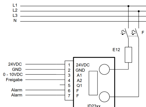
Abbildung 8: typischer Anschluss 400VAC
