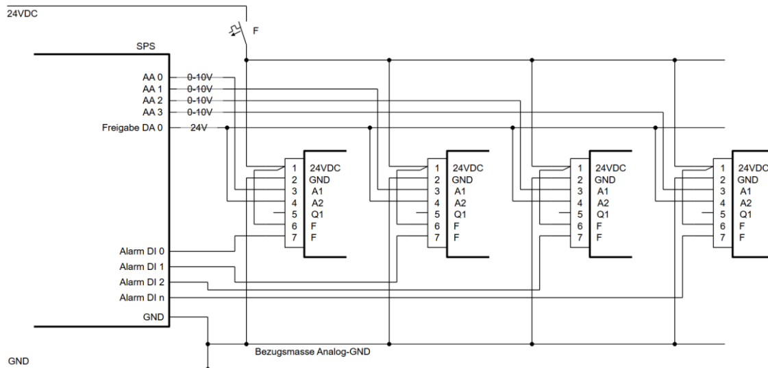
Abbildung 13: Ausführung mit Einzelalarm-Auswertung
