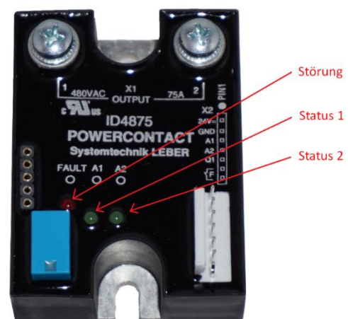
Abbildung 4: Status-LEDs
