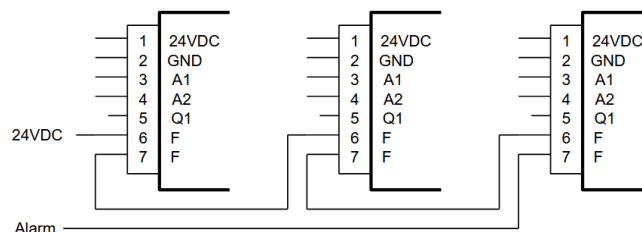
Abbildung 14: Ausführung mit Summen-Alarm-Auswertung
