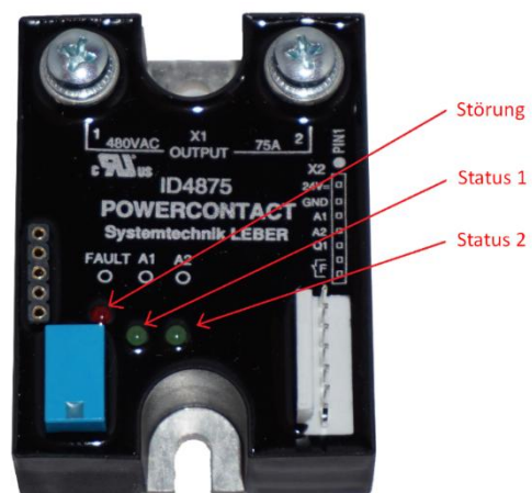
Abbildung 4: Status-LEDs
