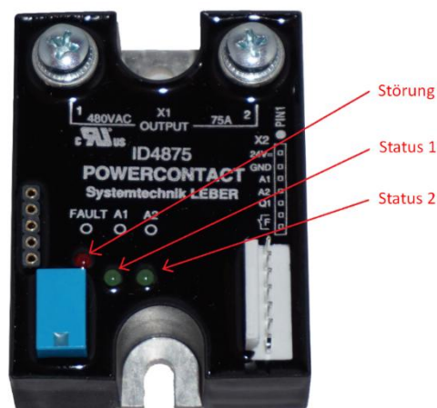
Abbildung 4: Status-LEDs
