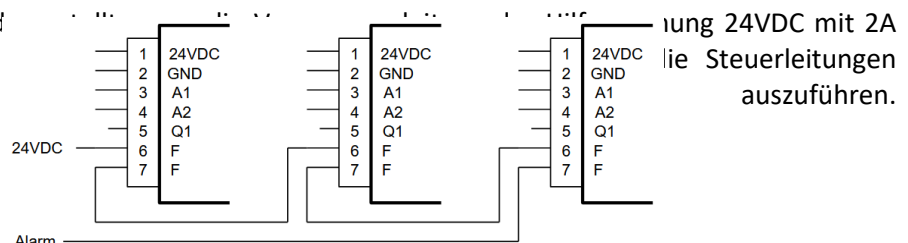
Abbildung 14: Ausführung mit Summen-Alarm-Auswertung
