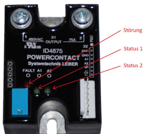
Abbildung 4: Status-LEDs
