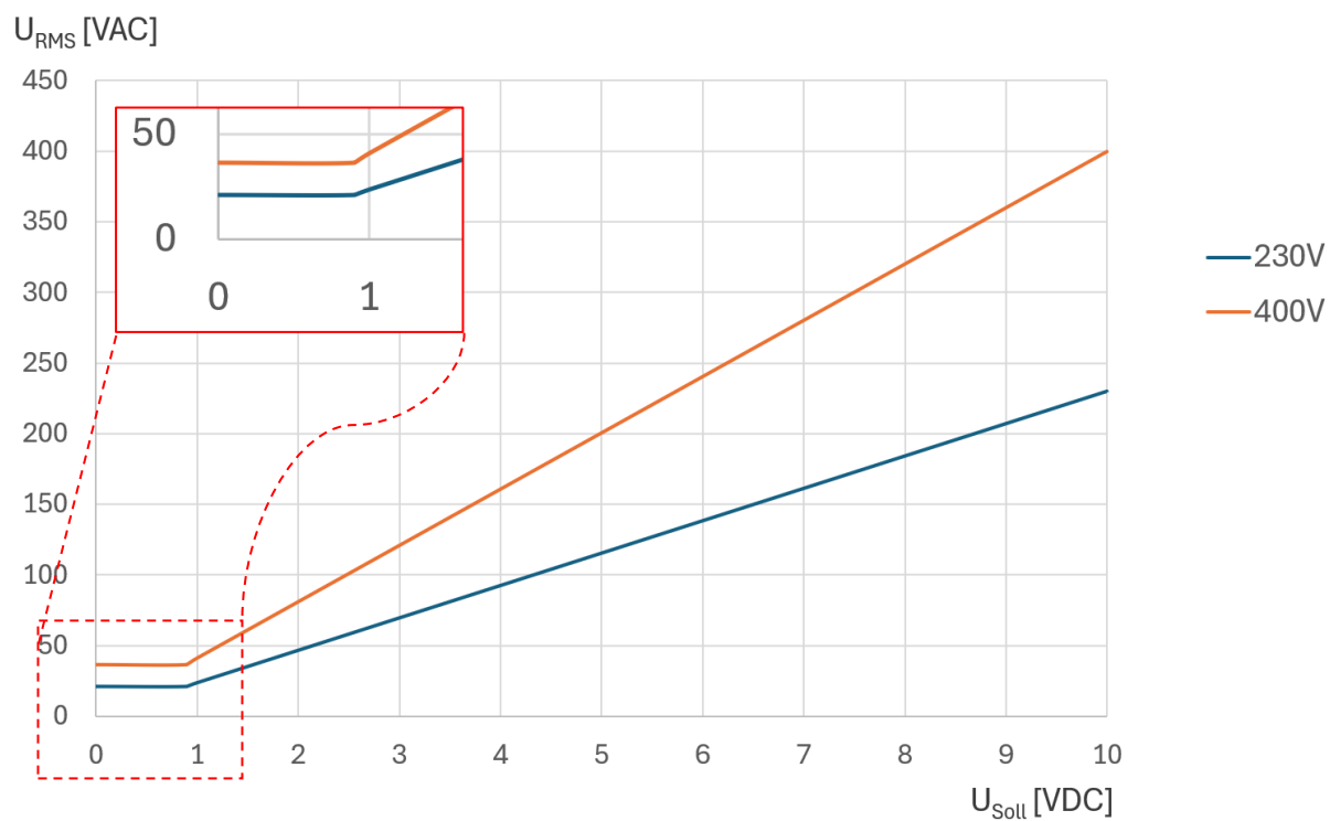
Abbildung 10: Effektive Lastspannung vs. Steuerspannung
