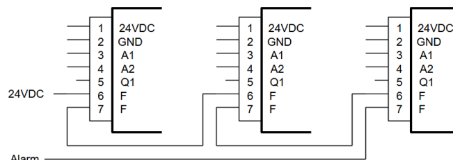
Abbildung 14: Auswertung mit Summen-Alarm-Auswertung
