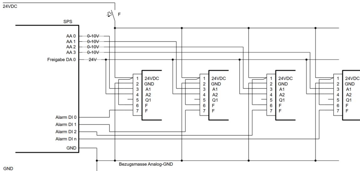
Abbildung 13: Ausführung mit Einzelalarm-Auswertung
