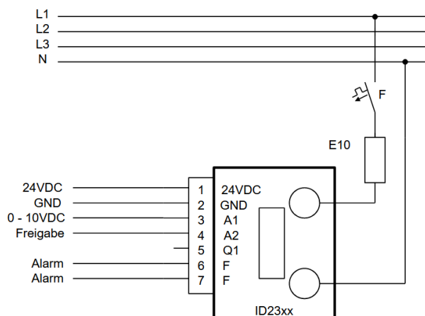
Abbildung 7: typischer Anschluss 230VAC
