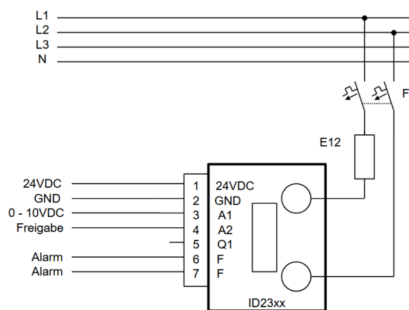
Abbildung 8: typischer Anschluss 400VAC
