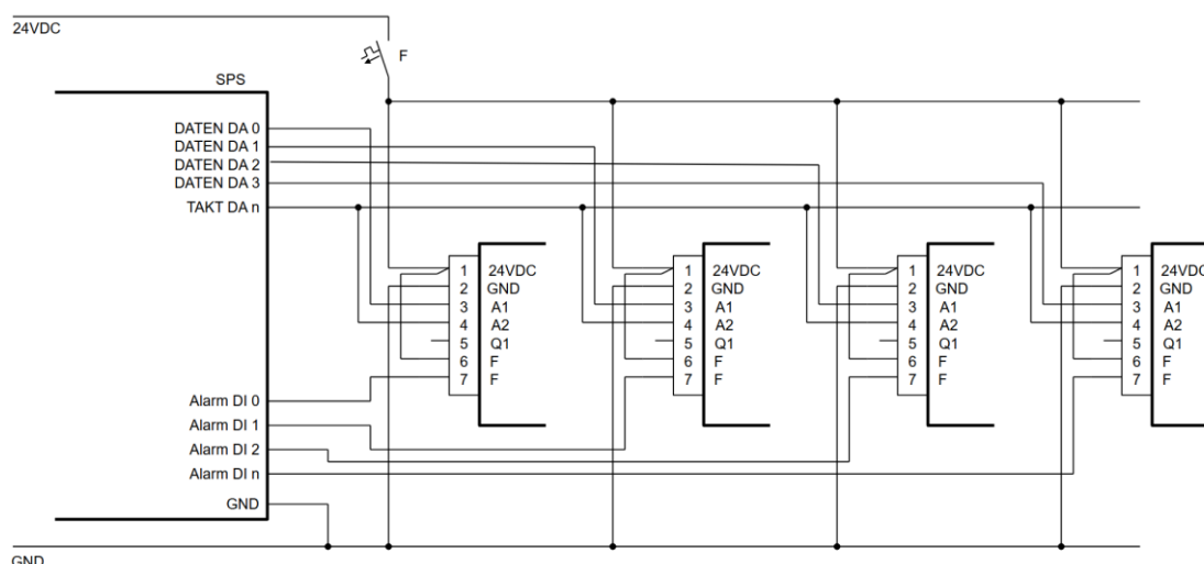
Abbildung 14: Ausführung mit Einzelalarm-Auswertung
