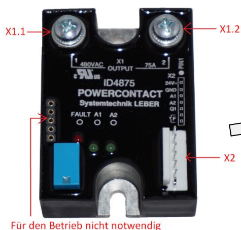
Abbildung 5: Belegung Stecker X1.1, X1.2 und X2
