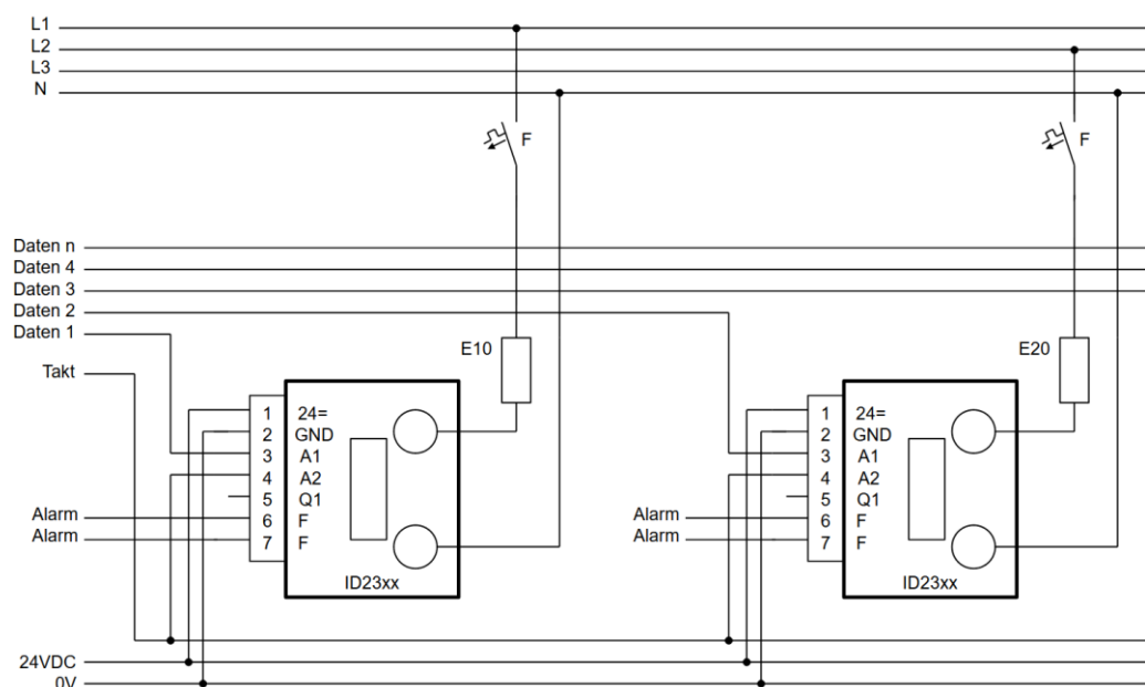
Abbildung 4: Steuerung mittels „TransDil-Protokolls“
