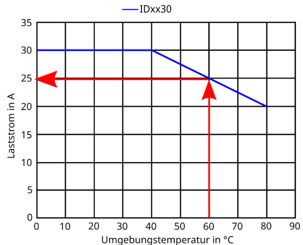
Abbildung 13: Beispiel zur Ermittlung des max. zulässigen Laststroms
