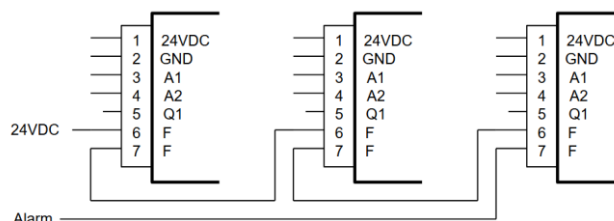
Abbildung 15: Ausführung mit Summen-Alarm-Auswertung
