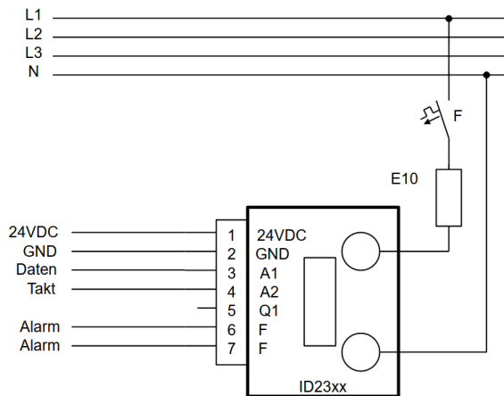
Abbildung 9: typischer Anschluss 230VAC
