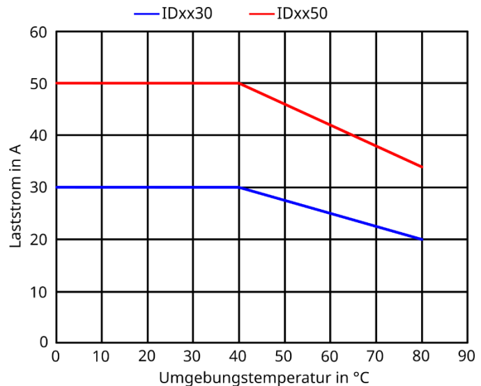
Abbildung 12: Derating Kurve für die Steller ID2330 und ID2350
