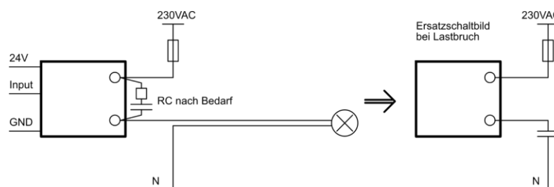
Abbildung 16: Kapazität parallel verlegter Kabel
