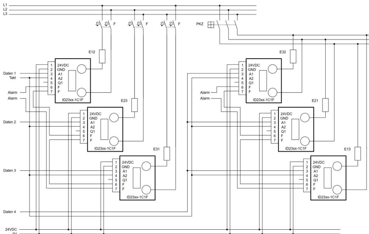
Abbildung 11: Darstellung von 3-phasen Anwendungen
