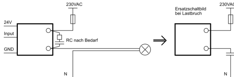
Abbildung 14: Kapazität parallel verlegter Kabel
