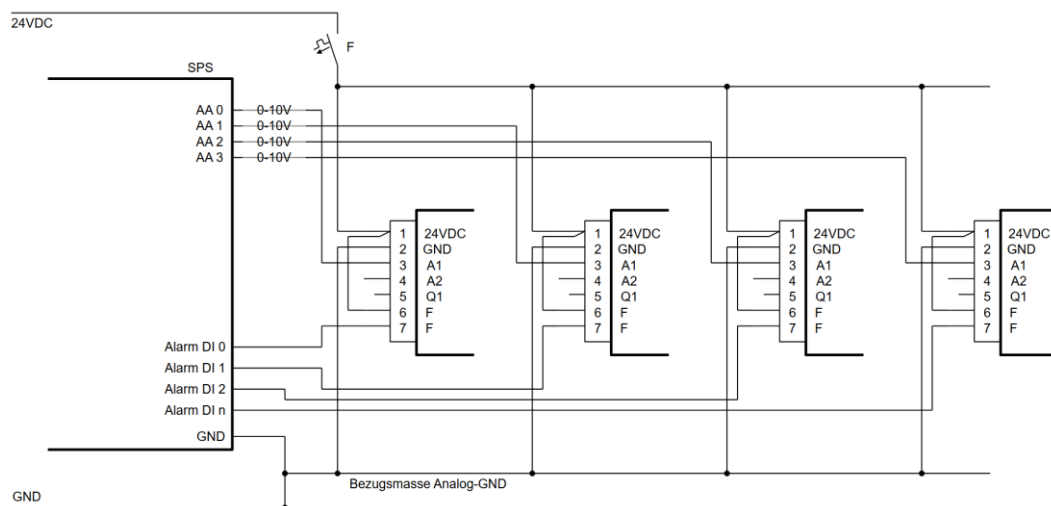
Abbildung 12: Ausführung mit Einzelalarm-Auswertung
