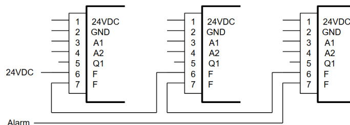
Abbildung 13: Ausführung mit Summen-Alarm-Auswertung
