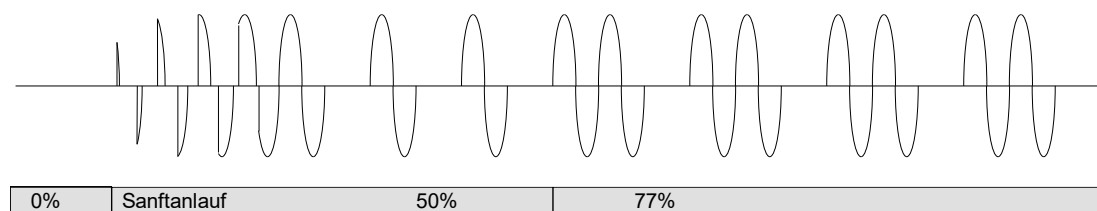
Abbildung 2: Darstellung der Vorheizphase & der Pulspakete bei verschiedenen Stellwerten
