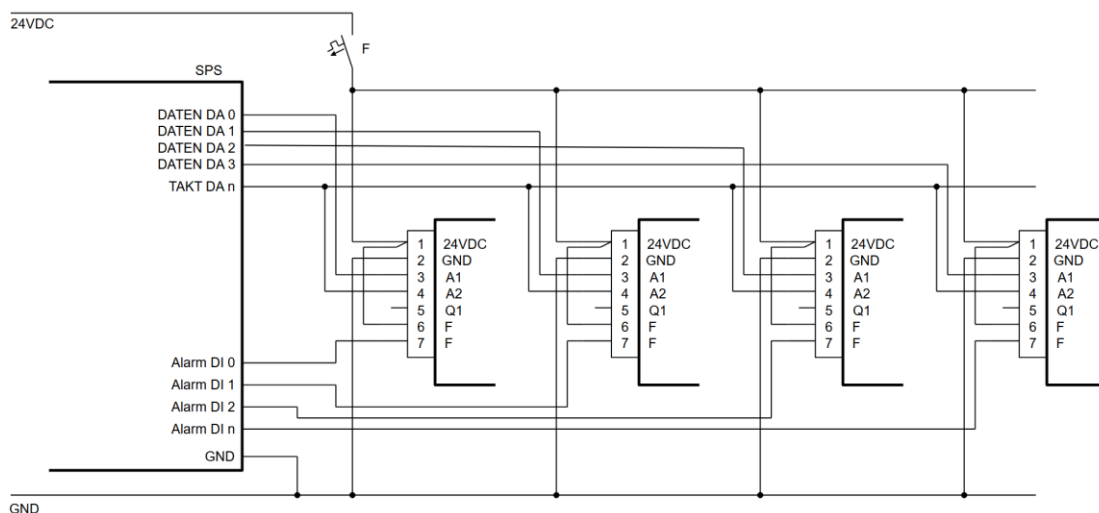
Abbildung 14: Ausführung mit Einzelalarm-Auswertung
