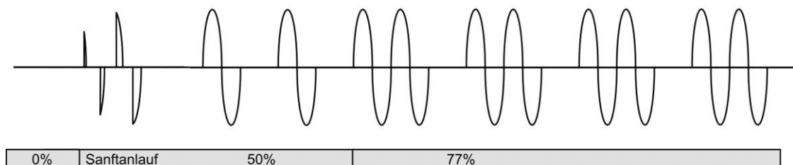
Abbildung 2: Darstellung der Pulspakete bei verschiedenen Stellwerten
