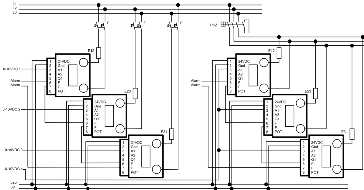
Abbildung 10: Darstellung von 3-phasen Anwendungen
