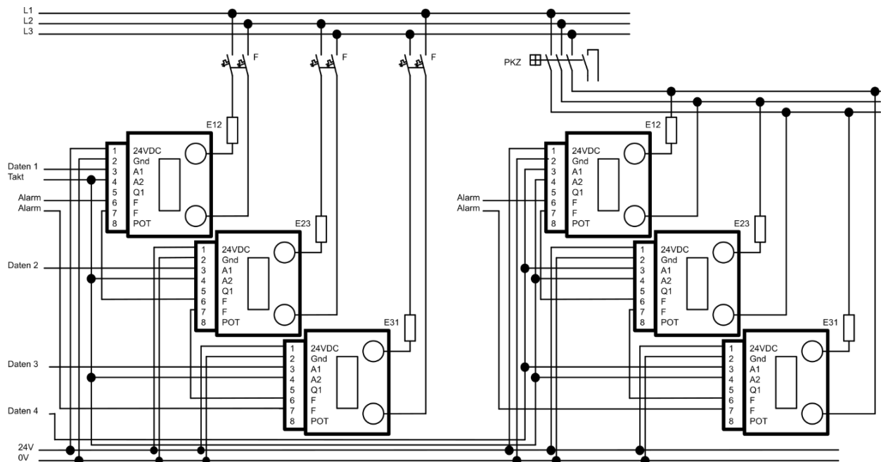
Abbildung 12: Darstellung von 3-phases Anwendungen
