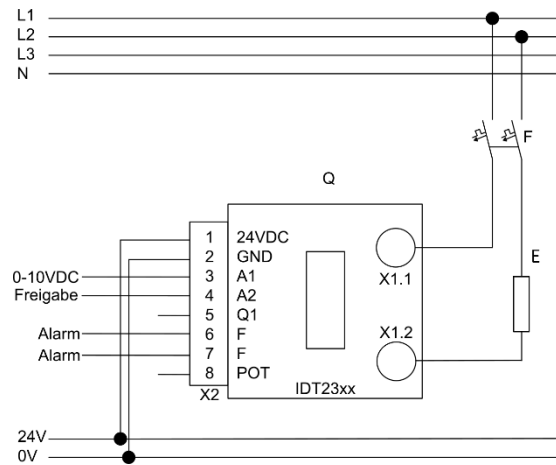
Abbildung 9: typischer Anschluss 400VAC
