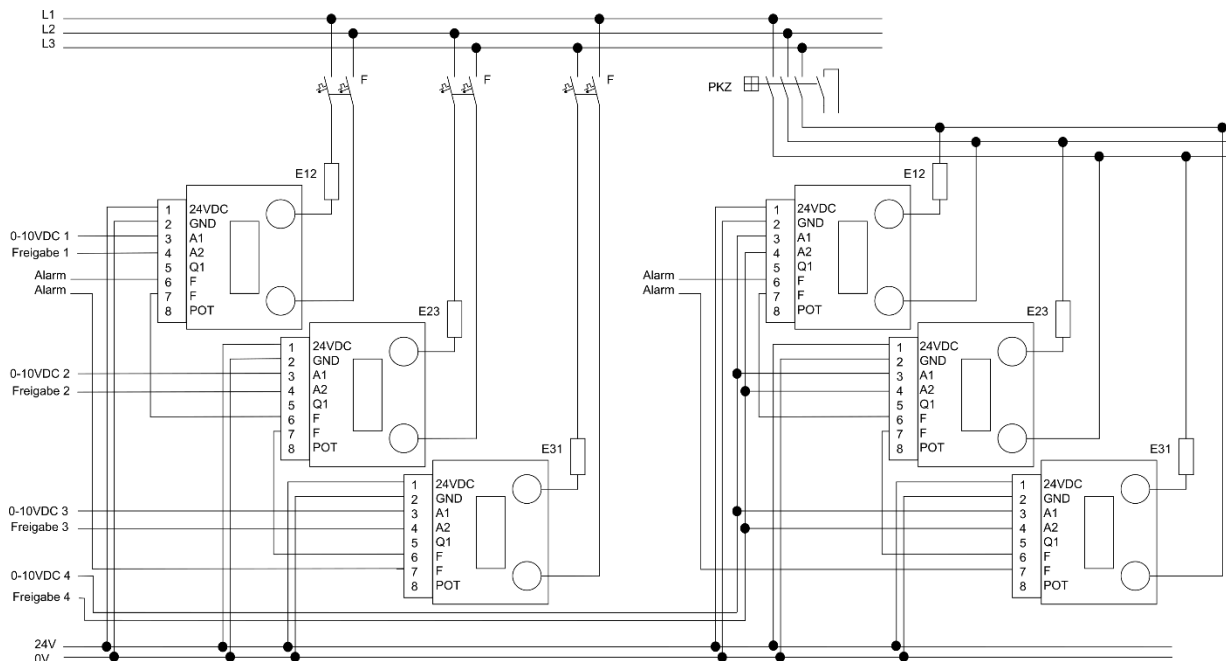
Abbildung 10: Darstellung von 3-phasen Anwendungen
