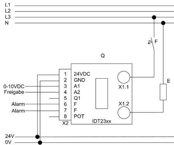
Abbildung 8: typischer Anschluss 230VAC
