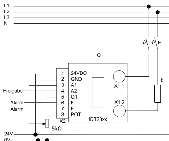
Abbildung 11: Ansteuerung mittels Potentiometer
