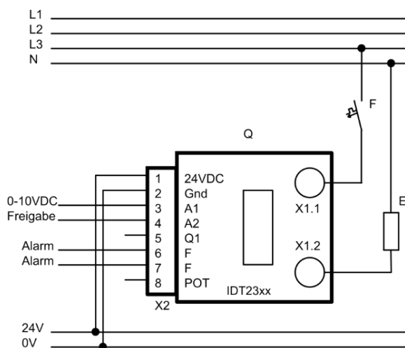
Abbildung 8: typischer Anschluss 230VAC
