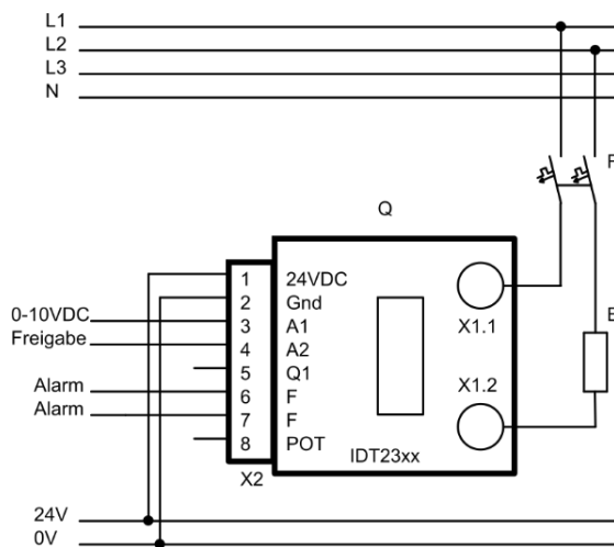
Abbildung 9: typischer Anschluss 400VAC
