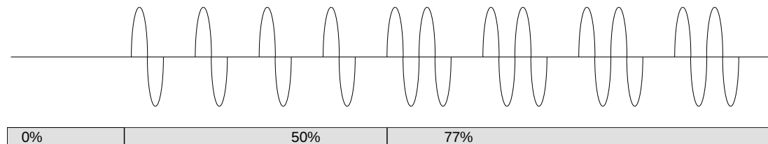
Abbildung 2: Darstellung der Pulspakete bei verschiedenen Stellwerten
