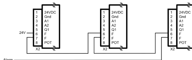
Abbildung 17: Ausführung mit Summen-Alarm-Auswertung
