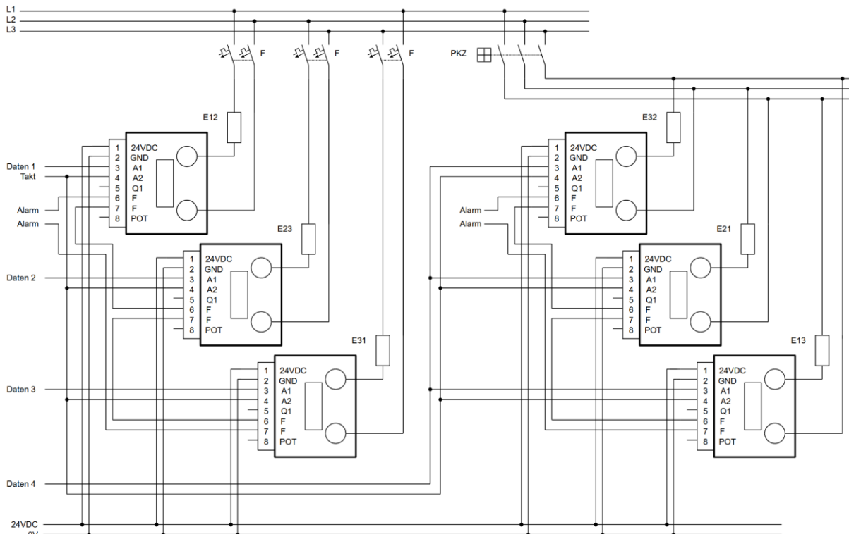
Abbildung 12: Darstellung von 3-phasen Anwendungen
