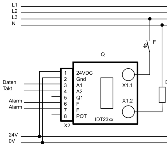
Abbildung 10: typischer Anschluss 230VAC
