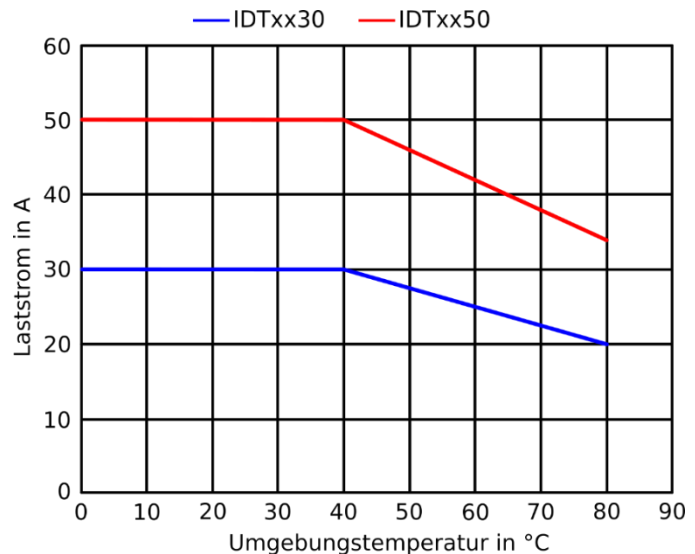
Abbildung 14: Derating Kurve für die Steller IDT2330 und IDT2350
