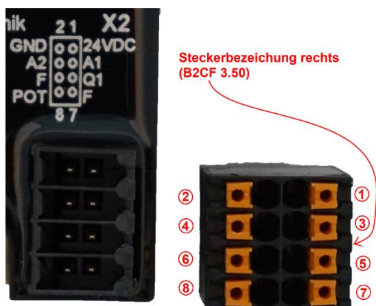
Abbildung 5: Belegung Stecker X2
