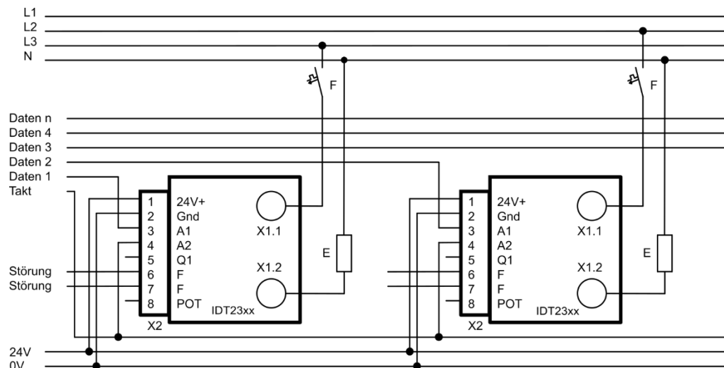
Abbildung 4: Steuerung mittels „TransDil-Protokolls“
