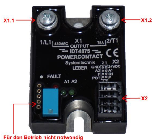
Abbildung 6: Leistungsanschlüsse X1.1 und X1.2
