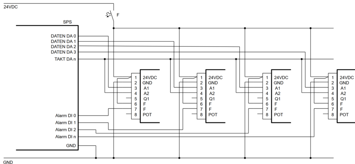
Abbildung 16: Ausführung mit Einzelalarm-Auswertung
