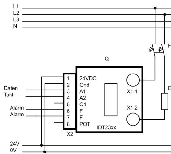
Abbildung 11: typischer Anschluss 400VAC
