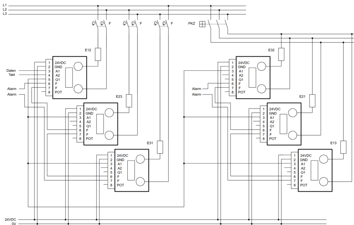
Abbildung 13: Darstellung von 3-phasen Anwendungen im Master-Slave-Betrieb
