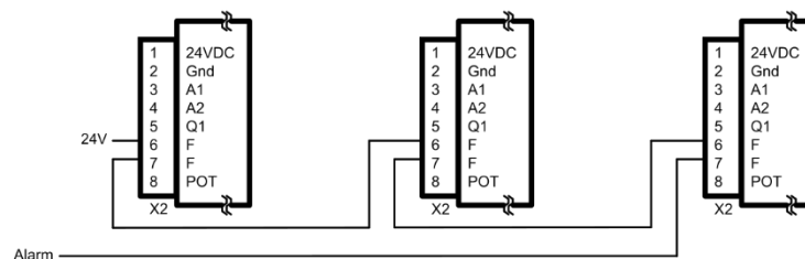
Abbildung 12: Ausführung mit Summen-Alarm-Auswertung
