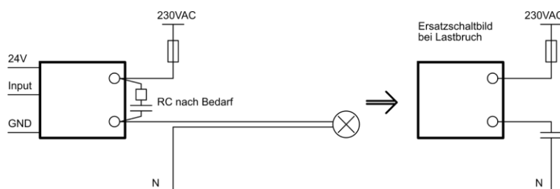
Abbildung 13: Kapazität parallel verlegter Kabel
