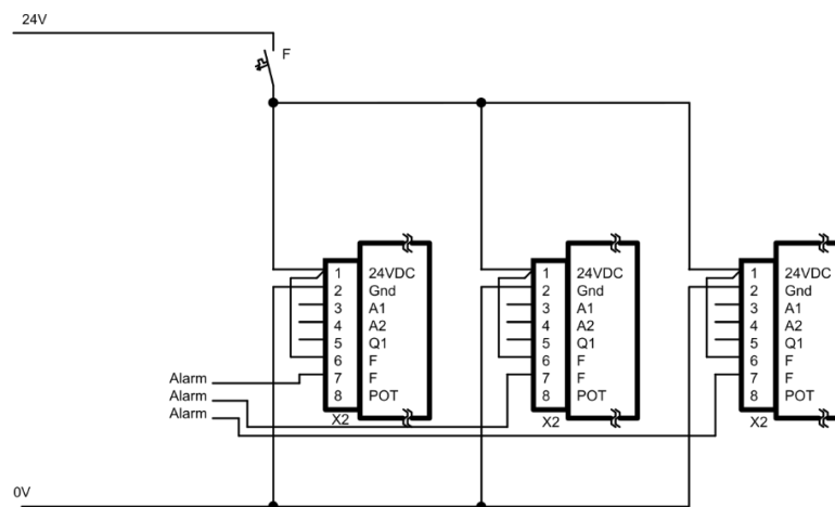
Abbildung 11: Ausführung mit Einzelalarm-Auswertung
