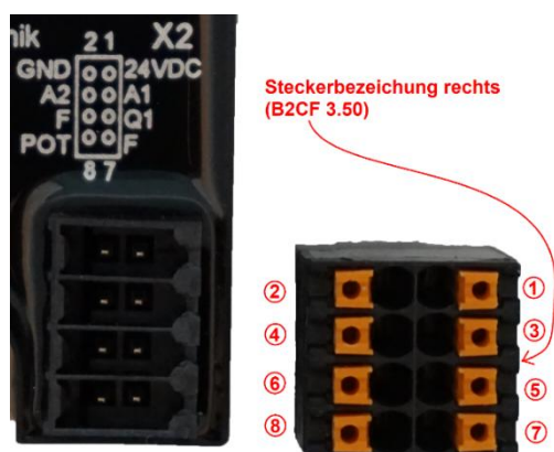
Abbildung 3: Belegung Stecker X2
